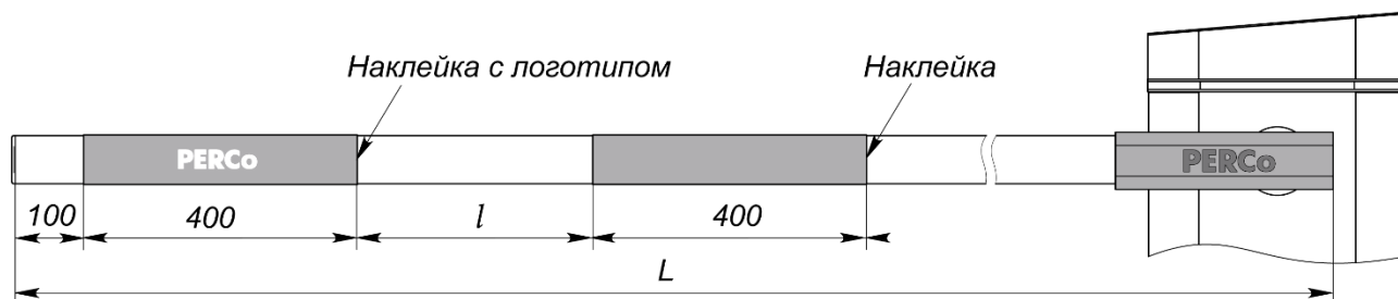
Рисунок 12. Наклеивание световозвращающих элементов на стрелу PERCo-GB0
