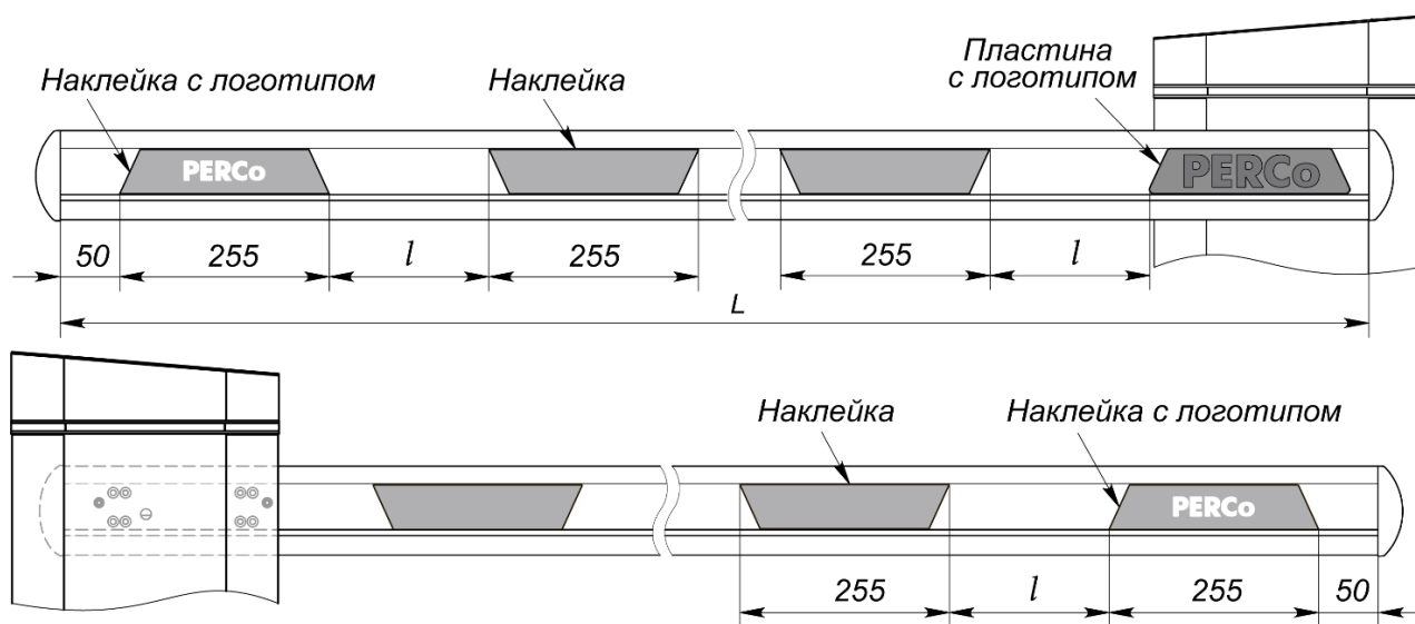
Рисунок 12. Наклеивание световозвращающих элементов на стрелу PERCo-GB0
