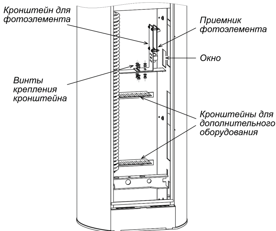
Рисунок 21. Установка фотоэлемента безопасности и доп. оборудования
